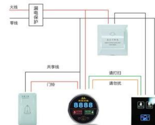
酒店客房/KTV/SPA会所 门牌房态显示门铃系统图
