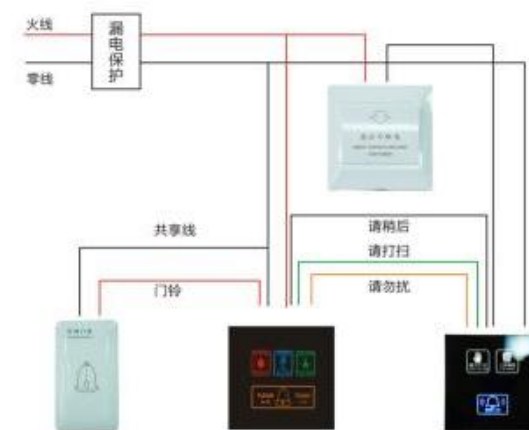
酒店会议室/KTV/公司办公室 房态显示门铃系统图
